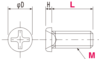
※0番1種形状 Type1-Driver size #0
