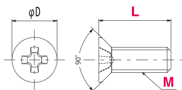
※0番1種形状 Type1-Driver size #0
