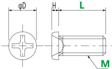
※0番1種形状 Type1-Driver size #0
